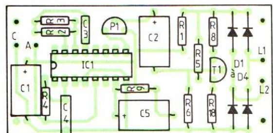
Fig. 3. - Implantation des composants.
