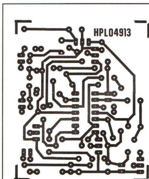
Fig. 2. - Circuit imprimé côté cuivre, échelle 1.
