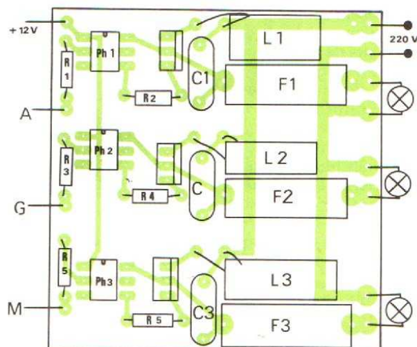
Fig. 3. - Implantation des composants.
