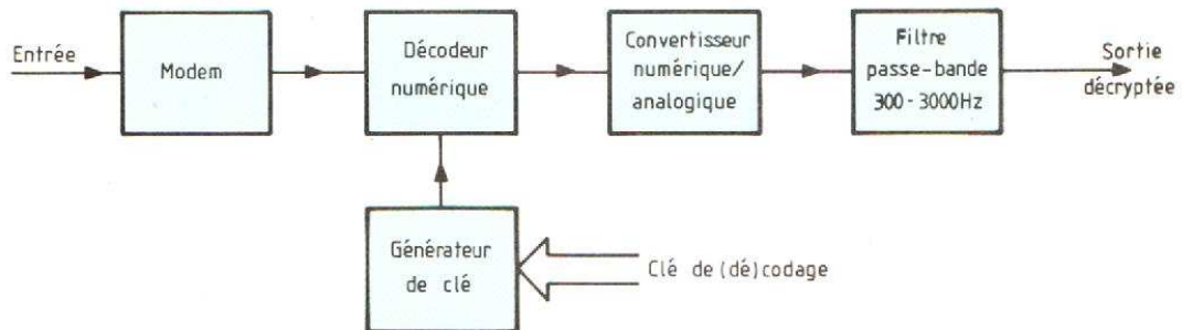
Fig. 4. Cryptophonie numérique : le décodeur.
