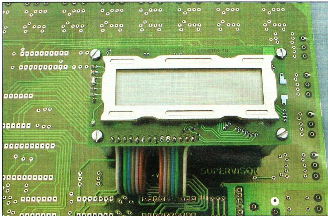
L'afficheur 2 lignes de 16 caractères à cristaux liquides.
