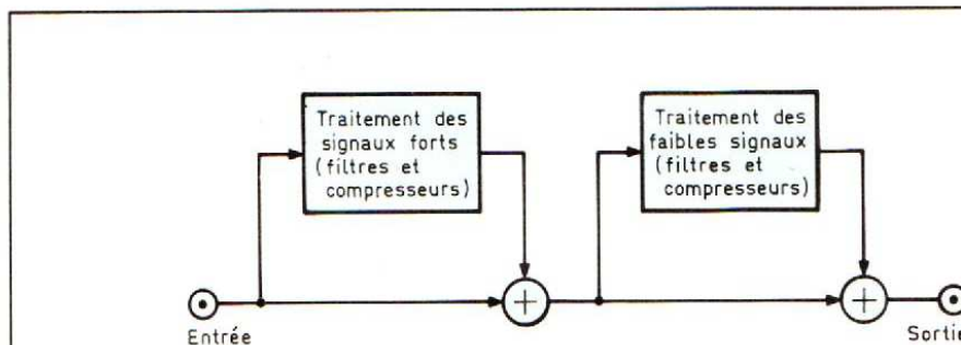
Fig. 3. - Principe du traitement décalé (en cascade) à deux niveaux : codage séparé des signaux forts, puis des signaux faibles (on le reconnaît aisément sur le synoptique de la fig. 1). Cette méthode, avec ses deux chaînes latérales successives, permet une compression supérieure du signal (jusqu'à 24 dB à certaines fréquences), sans perte de fiabilité au décodage. L'expérience montre que trop compresser, en une seule opération, est une opération souvent risquée.
