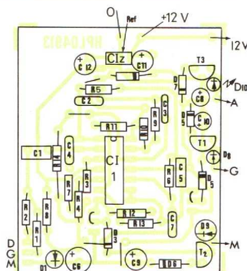
Fig. 3. - Implantation des composants.
