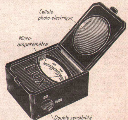
Fig. 2. — Luxmètre TUNGSRAM.
