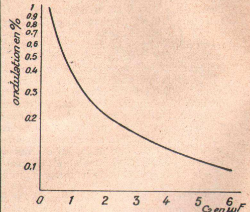
Fig. 5. — Variation de l'ondulation en fonction de la valeur du condensateur de sortie.
